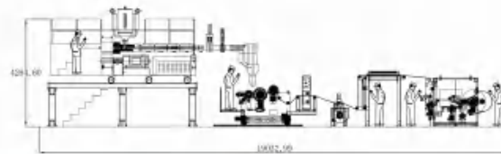
设备流程图 Flow chart
